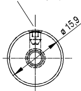
Gewindestifte M4 DIN916 A2 (2x)
